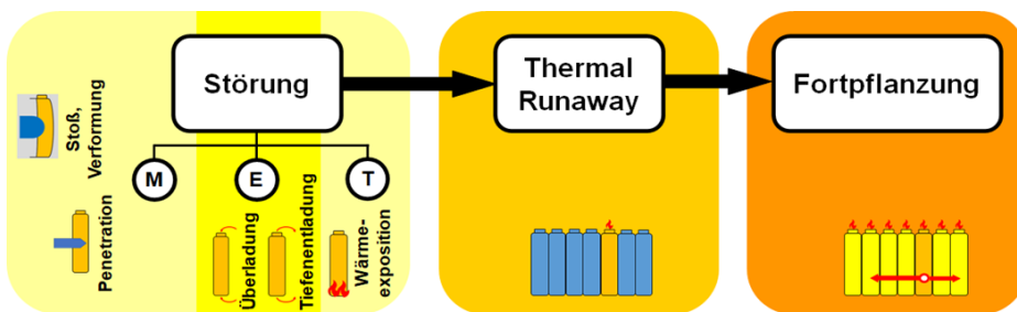
Abbildung 2: Beschreibung des Thermal Runaway
