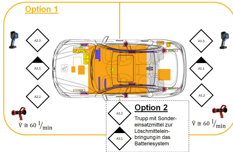
Abbildung 11: Empfehlung einer allgemeinen Vorgehensweise bei der Brandbekämpfung eines E-Fahrzeugs mit Beteiligung des Batteriesystems am Brand
