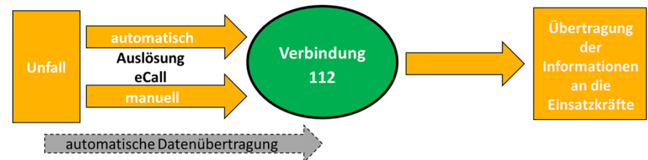
Abbildung 10: Prinzip von eCall
