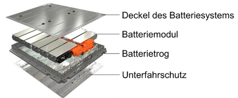
Abbildung 1: Batteriesystem mit Batteriegehäuse [3] mit Ergänzungen der Autoren
